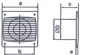
Maße - Skizze
